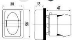
双位按钮 Double button
