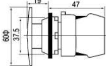
大头按钮 Big button
